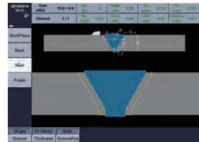
Ввод параметров шва объекта контроля
