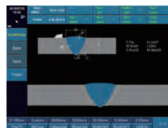
Односторонний V-шов
