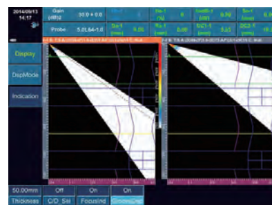
Построение разделки
