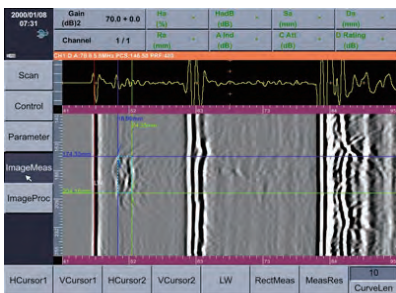
TOFD измерения
